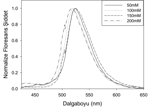
Şekil 10. Değişik tuz derişimlerinde kalıplanmış jelle piranin difüzyonu sonunda jelden alınan floresans spektrumları (uyarma dalgaboyu 400 nm'dir)
