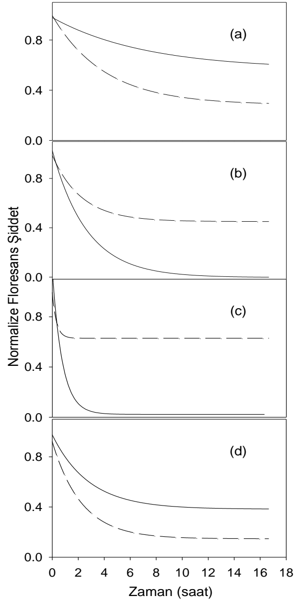
Şekil 4. İçinde aynı ölçü ve miktarlarda K1 ve R1 jeli bulunan değışik pıranin derişimlerinde floresans şiddetlerinin zamanla değışimi (Pıranin derişimleri: (a)= 10^{-5}M , (b)= 5 \times 10^{-6}M , (c)= 10^{-6}M , (d)= 5 \times 10^{-7}M )
